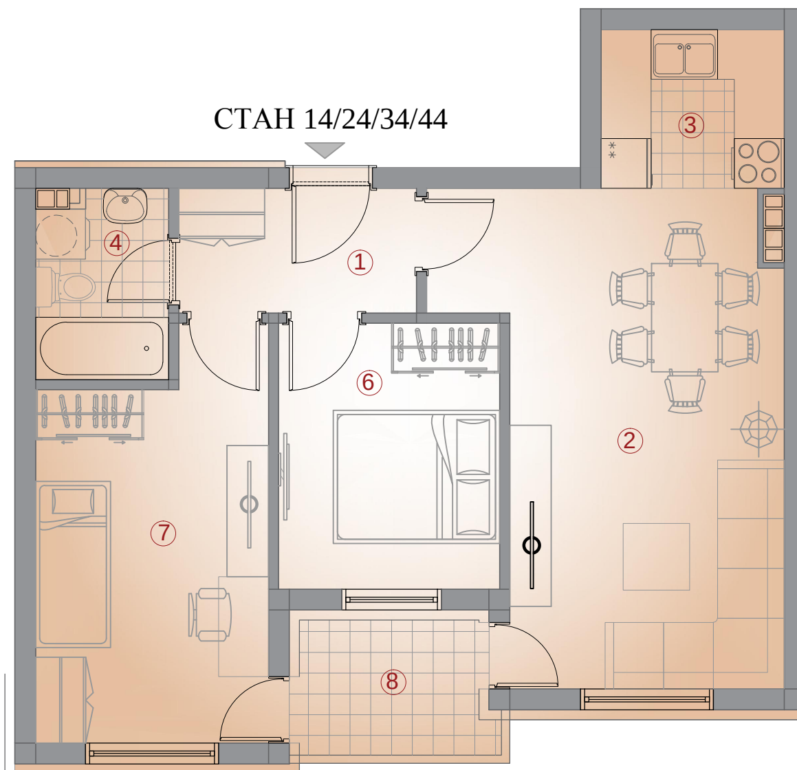
СТАН 14/24/34/44 - I,II,III,IV СПРАТ
