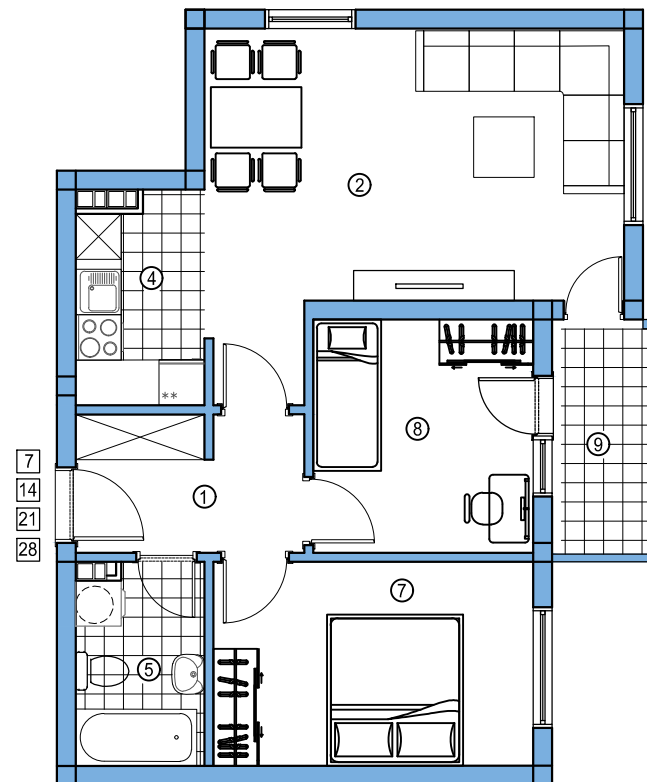
СТАН 7,14, 21 и 28 - I, II, III и IV СПРАТ (ламела 1)
