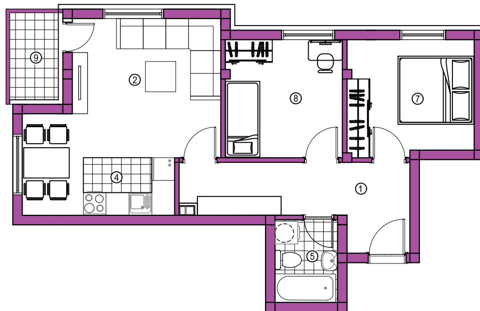
СТАН 6, 13, 22 и 27 - I, II, III и IV СПРАТ (ламела 1)
