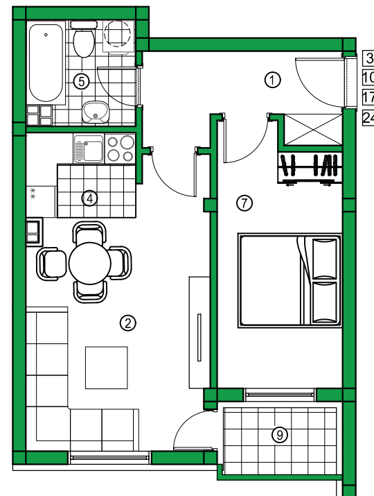
СТАН 3, 10, 17 и 24 - I, II, III и IV СПРАТ (ламела 1)
